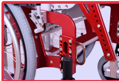
Befestigungsöse für Sicherung im Auto
