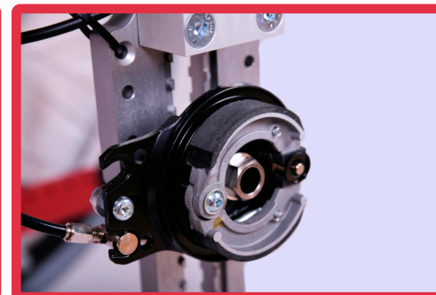
Trommelbremsrad 20" / 22" / 24"
