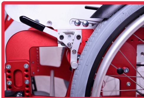
Kniehebelbremse
