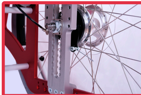
Sitzhöhenverstellung
